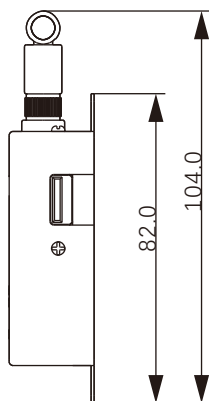
右视图
